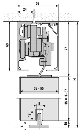
Deckenmontage
