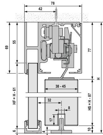
Deckenmontage mit Festflügel
