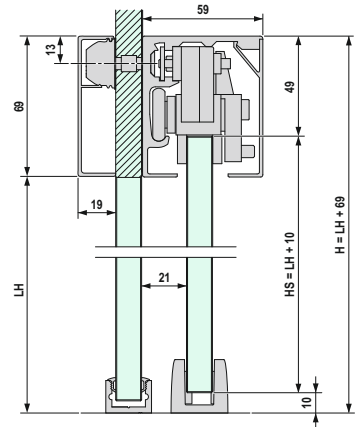
Glaswandmontage
