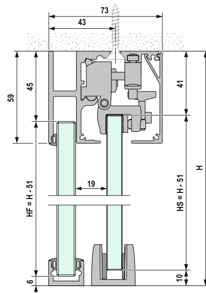
Deckenmontage mit Festflügel
