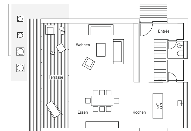
Geschlossen oder geöffnet: Mit einer Balkonschiebewand BSW wirken Garten und Wohnzimmer wie ein kompletter Raum.
