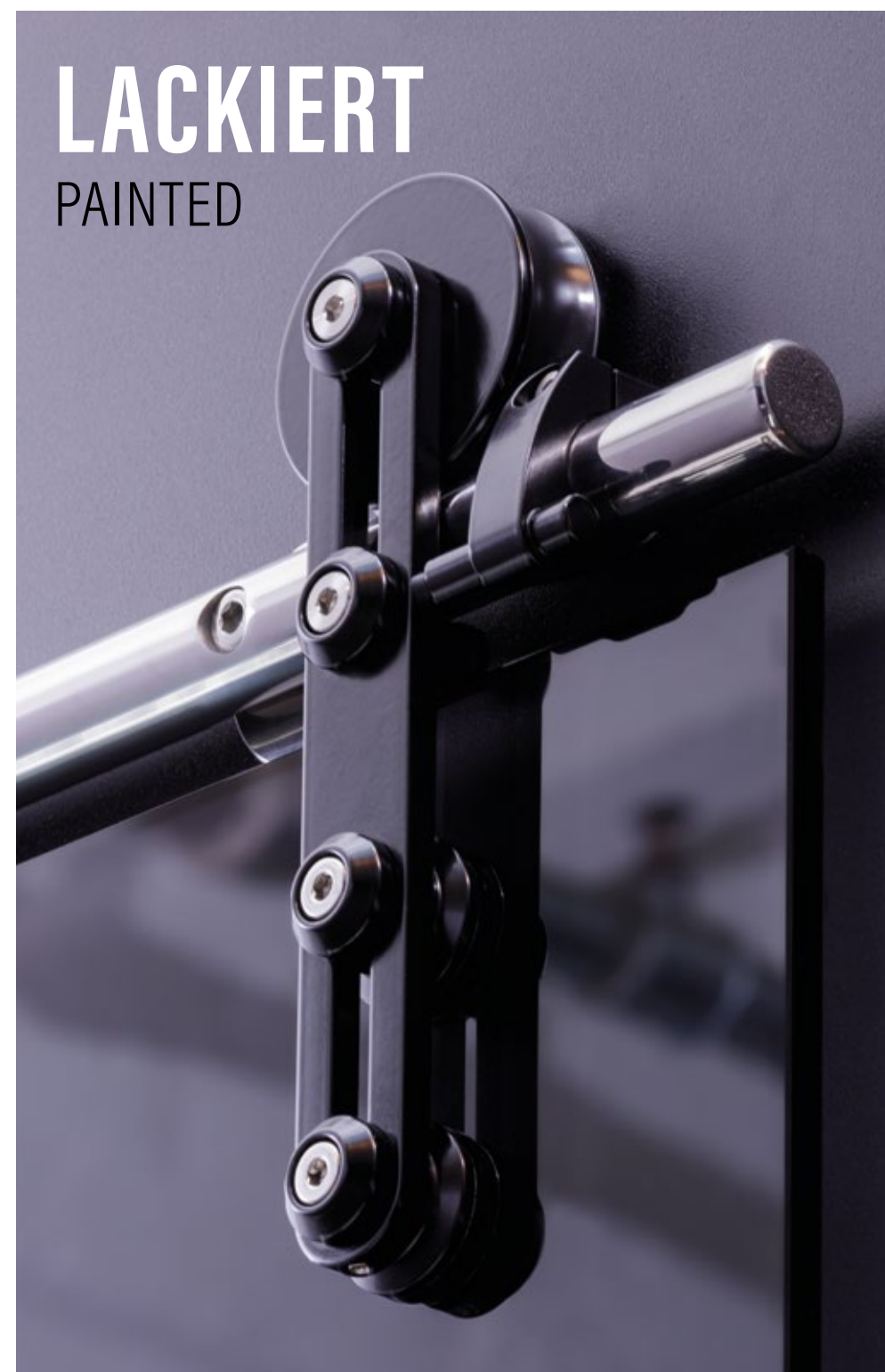
Türsystem ProTec, Rollwagen lackiert, Schrauben und Laufschiene Hochglanz spiegelpoliert door system ProTec, cart painted, screws and rail mirror polished
