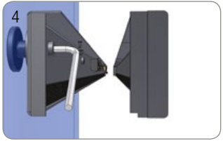
Glasbefestigung für 2-tlg. Führungsprofil | Glass fastener for 2-part guide profile
